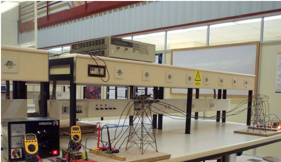
Figura 8: Prototipo de demostración del ahorro de energía en la transmisión a alta tensión.
