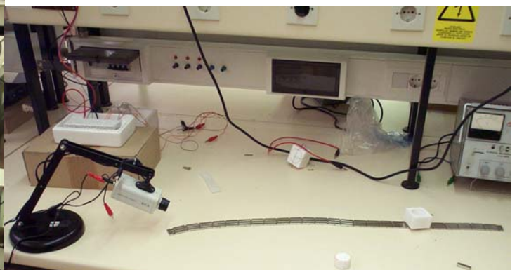
Figura 4: Superconductor levitado y cámara, al fondo izquierda se observa otro experimento con superconductores
