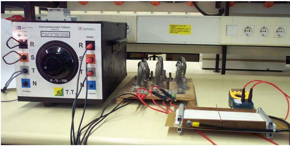
Figura 5: Prototipo para demostración de la fuerza de Lorentz. Consiste de una varilla móvil por la que circula una corriente, en presencia de un campo magnético.
