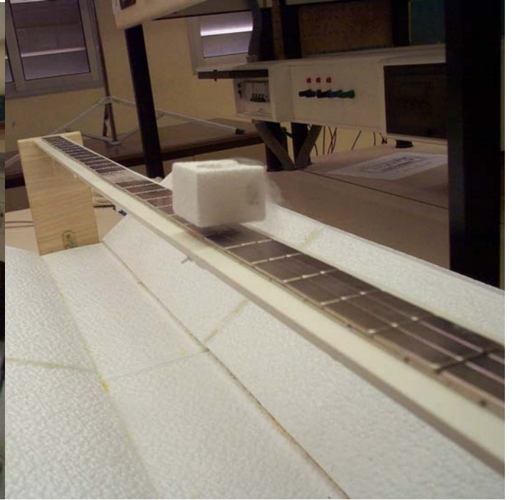
Figura 2: Detalle de superconductor levitado
