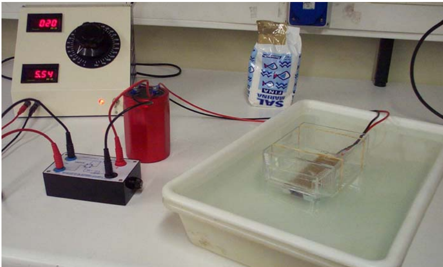
Figura 6: Prototipo para demostración de la fuerza de Lorentz para impulsar objetos en fluidos
