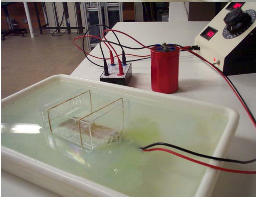
Figura 7: Detalle del prototipo anterior en funcionamiento.
