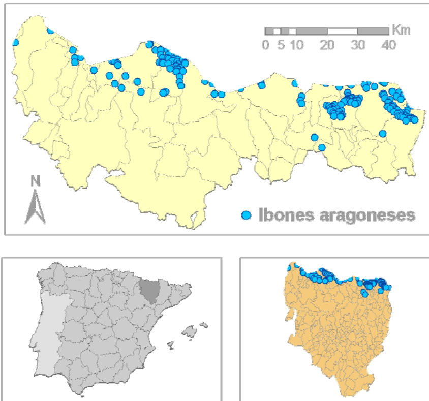
Fig. 2. Distribución del conjunto de lagos de alta montaña del Pirineo Aragonés (Datos de origen: CHE, 2009 y SITAR, 2009; Fuente: elaboración propia)
